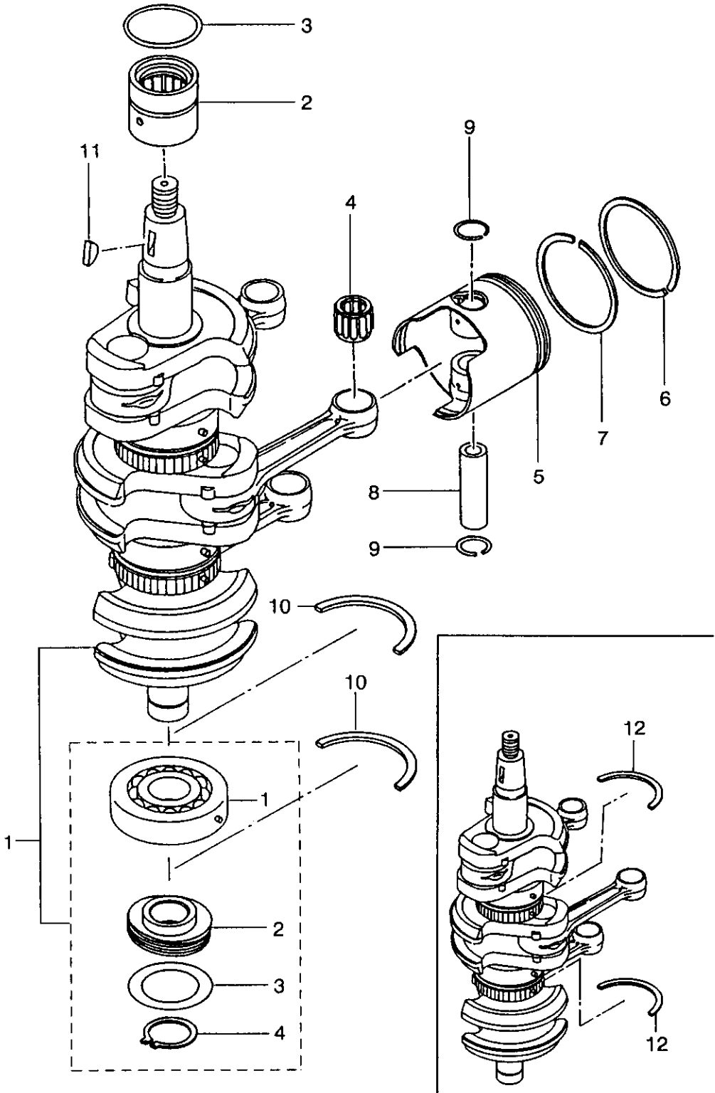
FIG. 2-A PISTON, CRANKSHAFT
