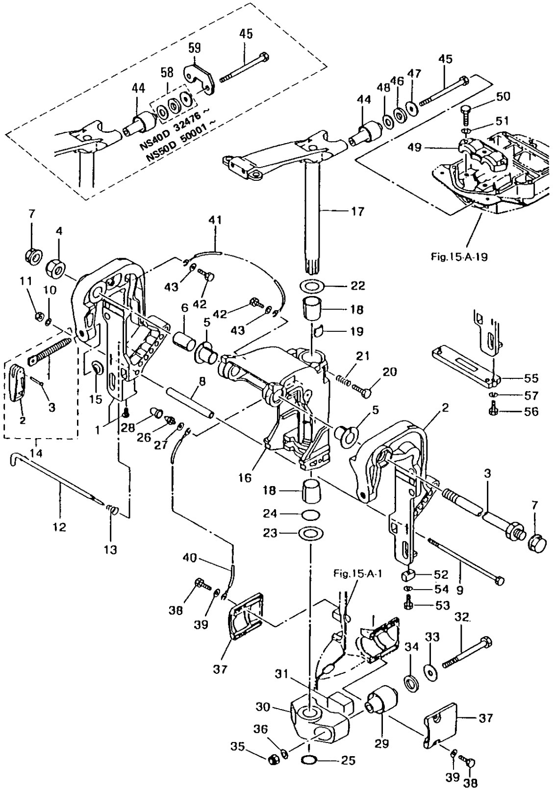
FIG. 19-A BRACKET
